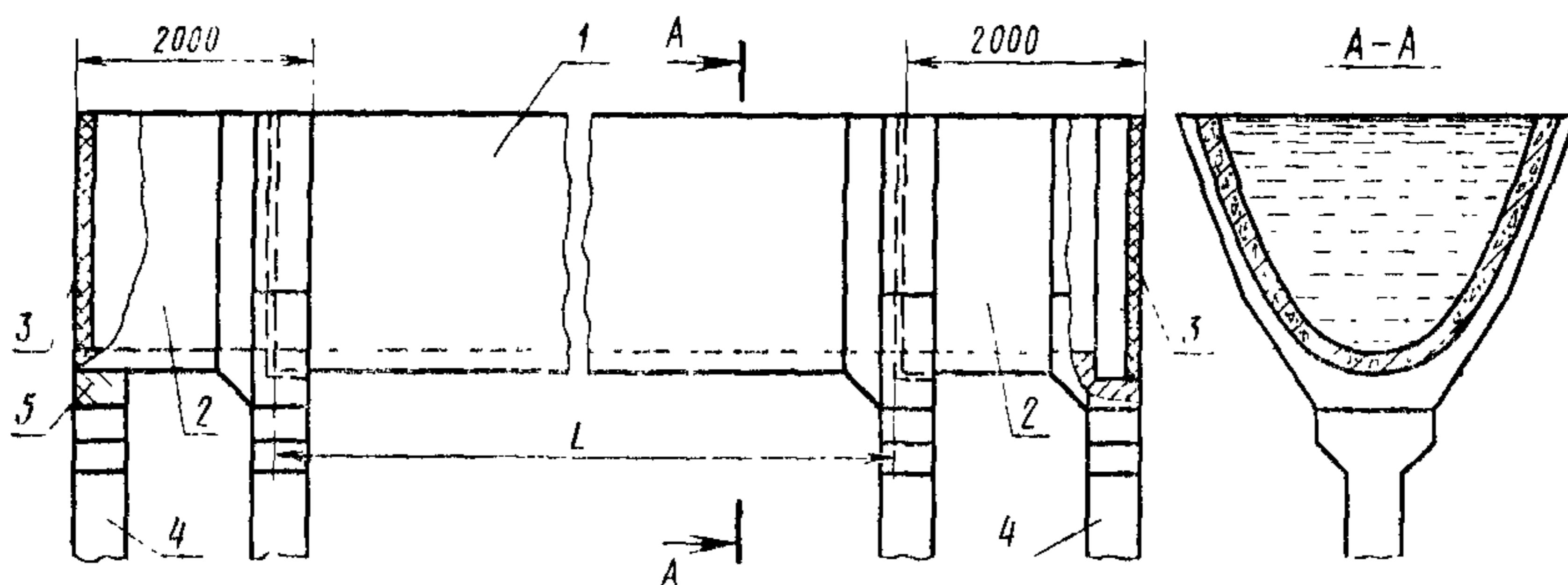
Схема гидростатических испытаний лотка на водонепроницаемость
